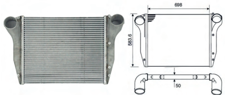
L1630/1635/1935/1941
