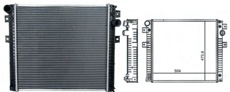
ACCELO 815/915 - S/L
